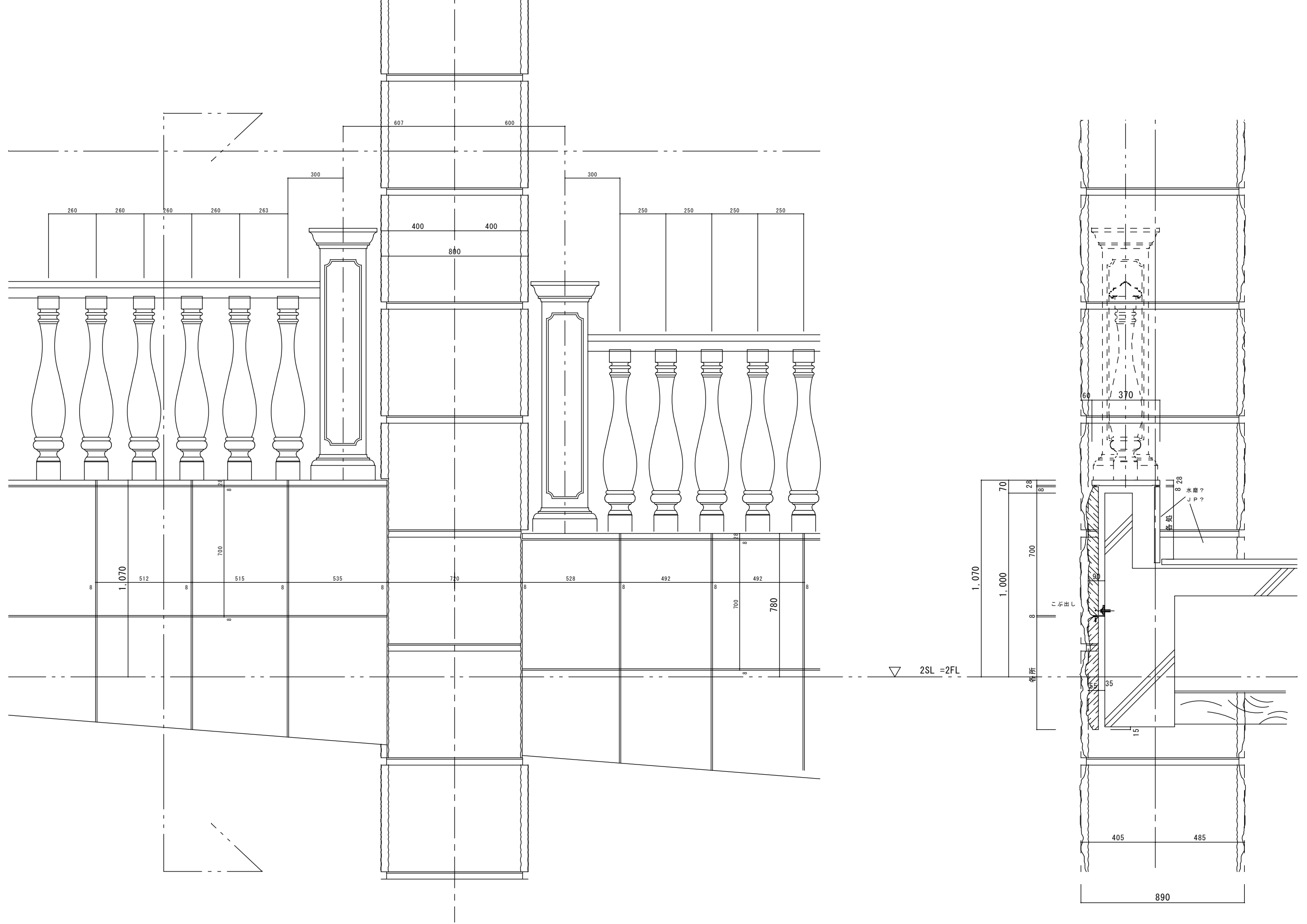
A-A断面図 1/10
